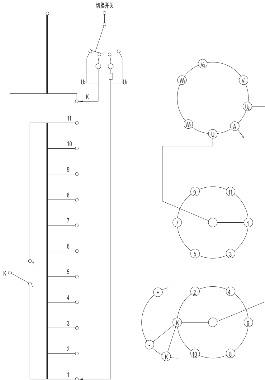
附图 28 SDZV 型有载分接开关 12233W 工作位置表和接线原理图
