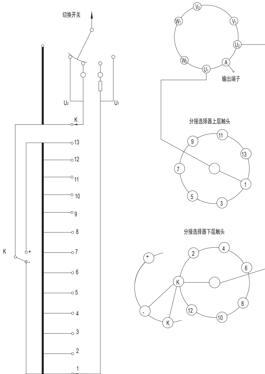
附图 31 SDZV 型有载分接开关 14273W 工作位置表和接线原理图
