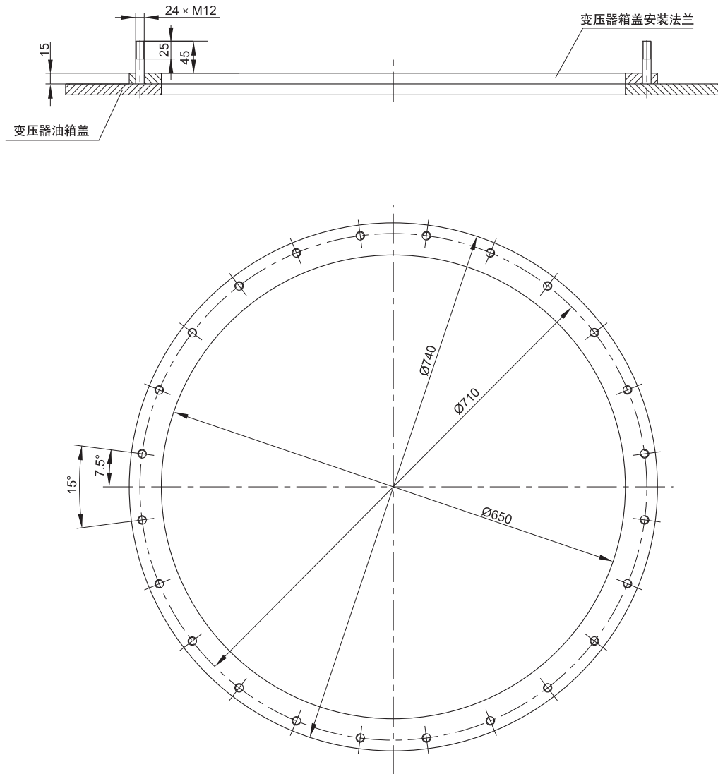
图-3 用于固定开关的法兰
