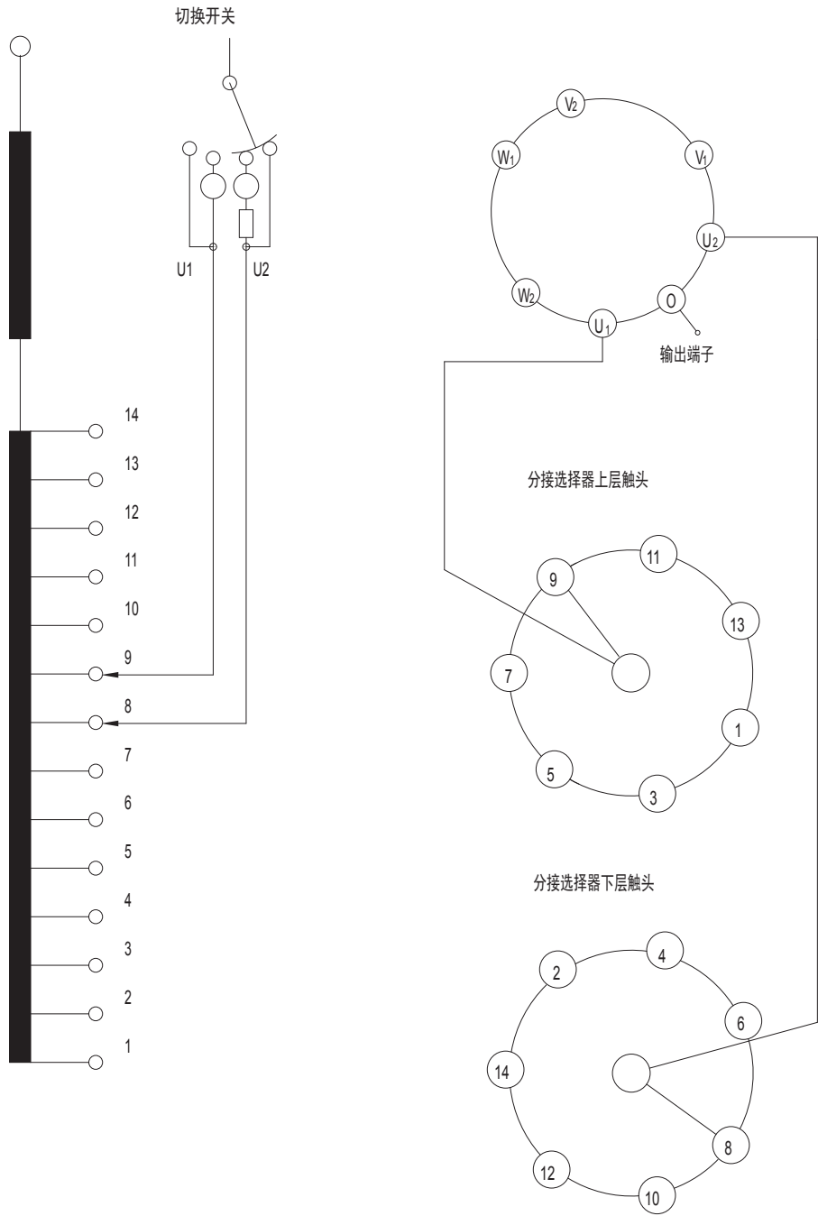
附图 17 SDZV 型有载分接开关 14140 工作位置表和接线原理图
