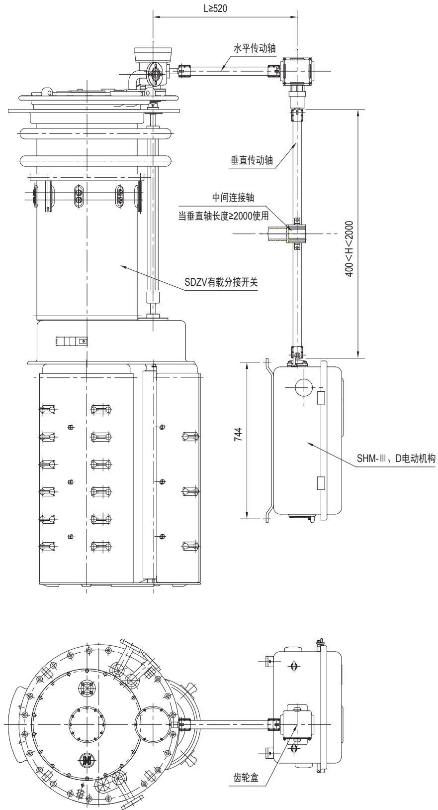
附图 8 SDZV 分接开关与 SHM电动机机构连接布置图
