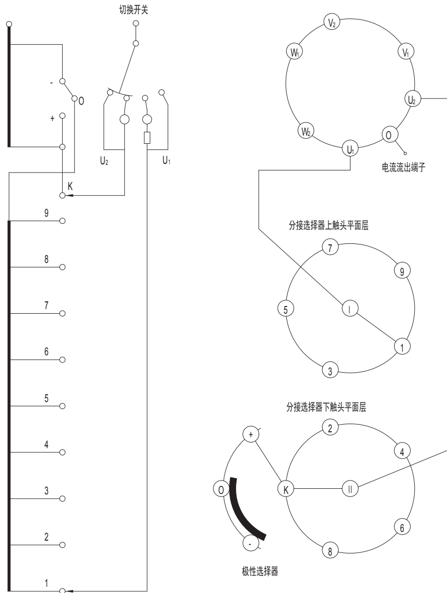
附图 24 SDZV 型有载分接开关 10193G 工作位置表和接线原理图
