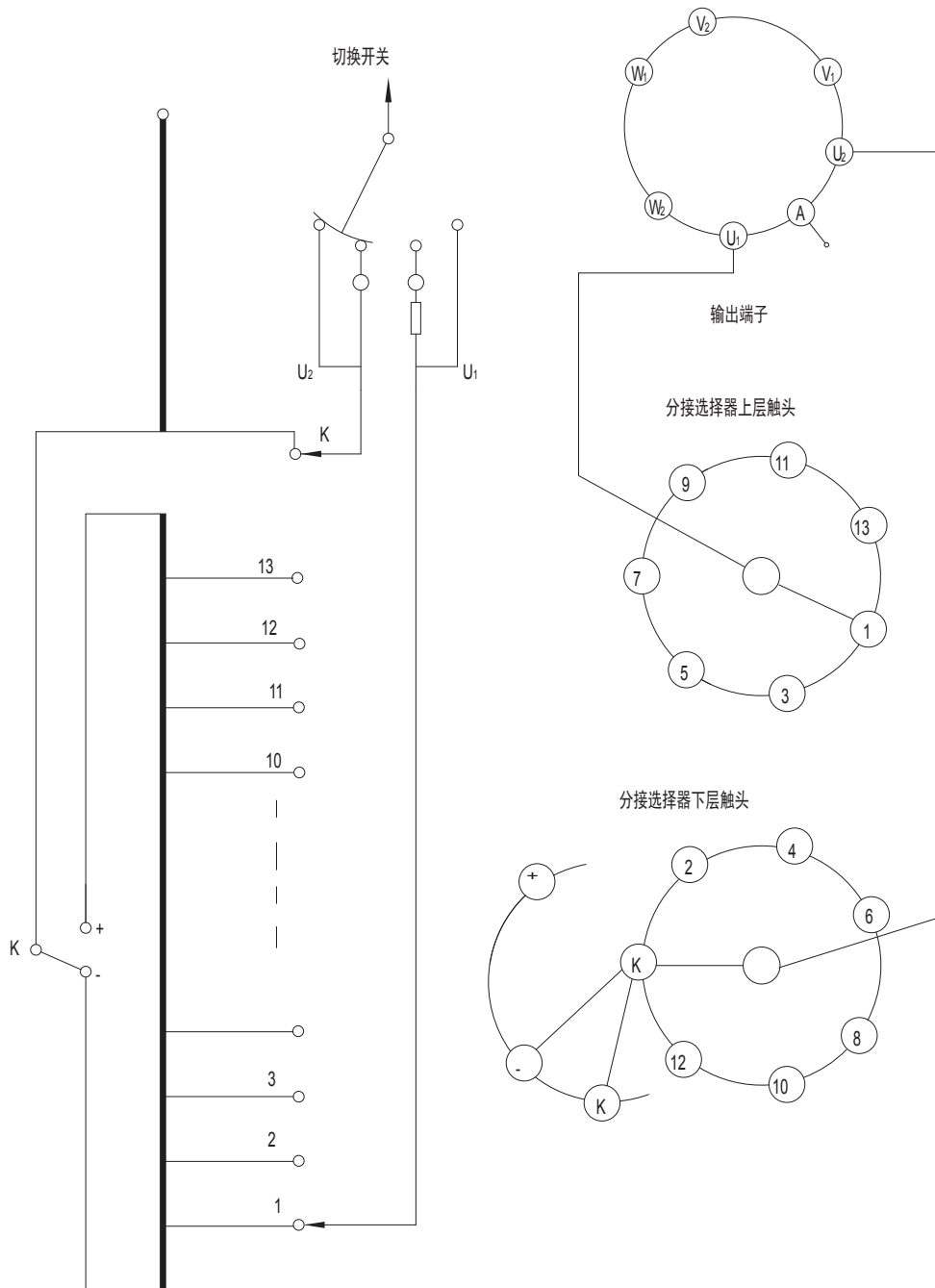
附图 30 SDZV 型有载分接开关 14271W 工作位置表和接线原理图
