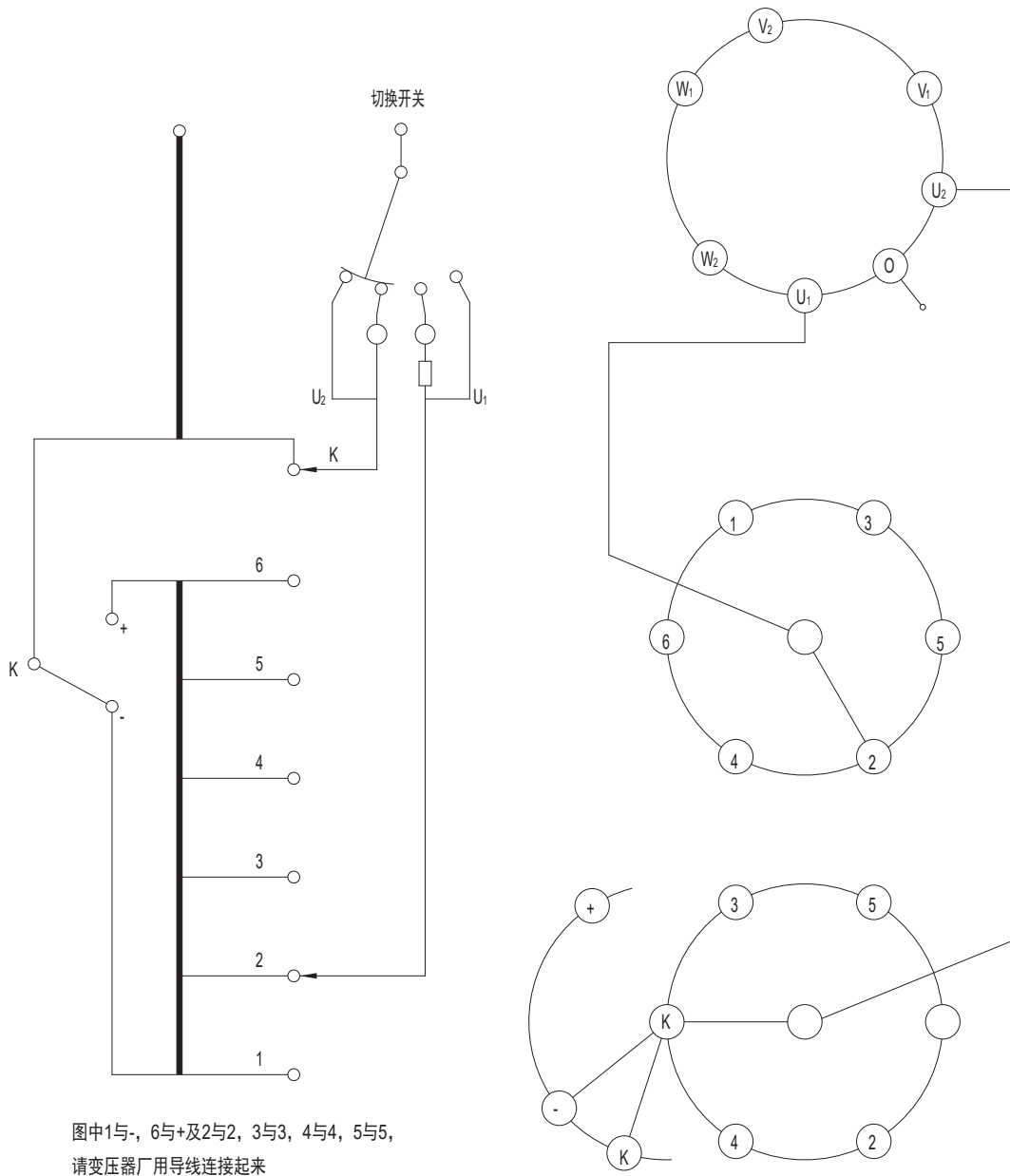
附图 25 SDZV 型有载分接开关 12111W 工作位置表和接线原理图
