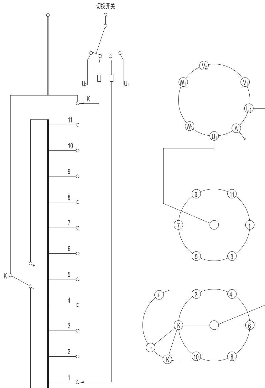
附图 26 SDZV 型有载分接开关 12231W 工作位置表和接线原理图
