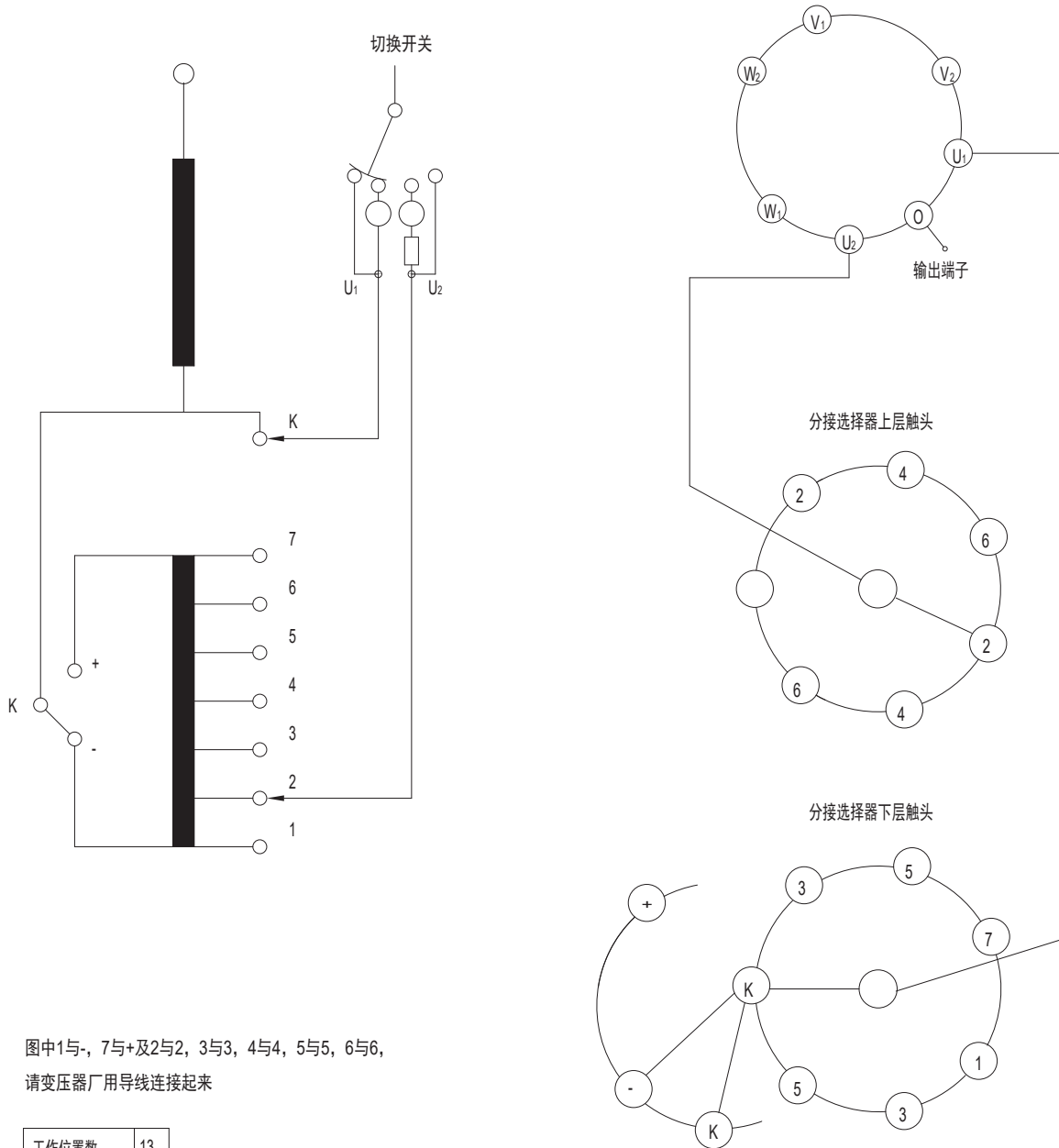
附图 29 SDZV 型有载分接开关 14131W 工作位置表和接线原理图
