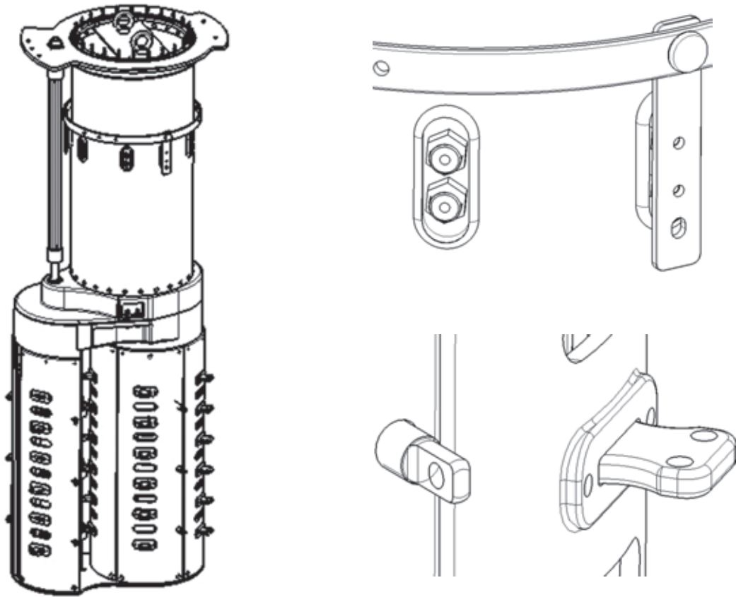
图-12 分接选择器和切换开关油室单双数导线连接
