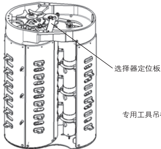
图-9 选择器定位板
