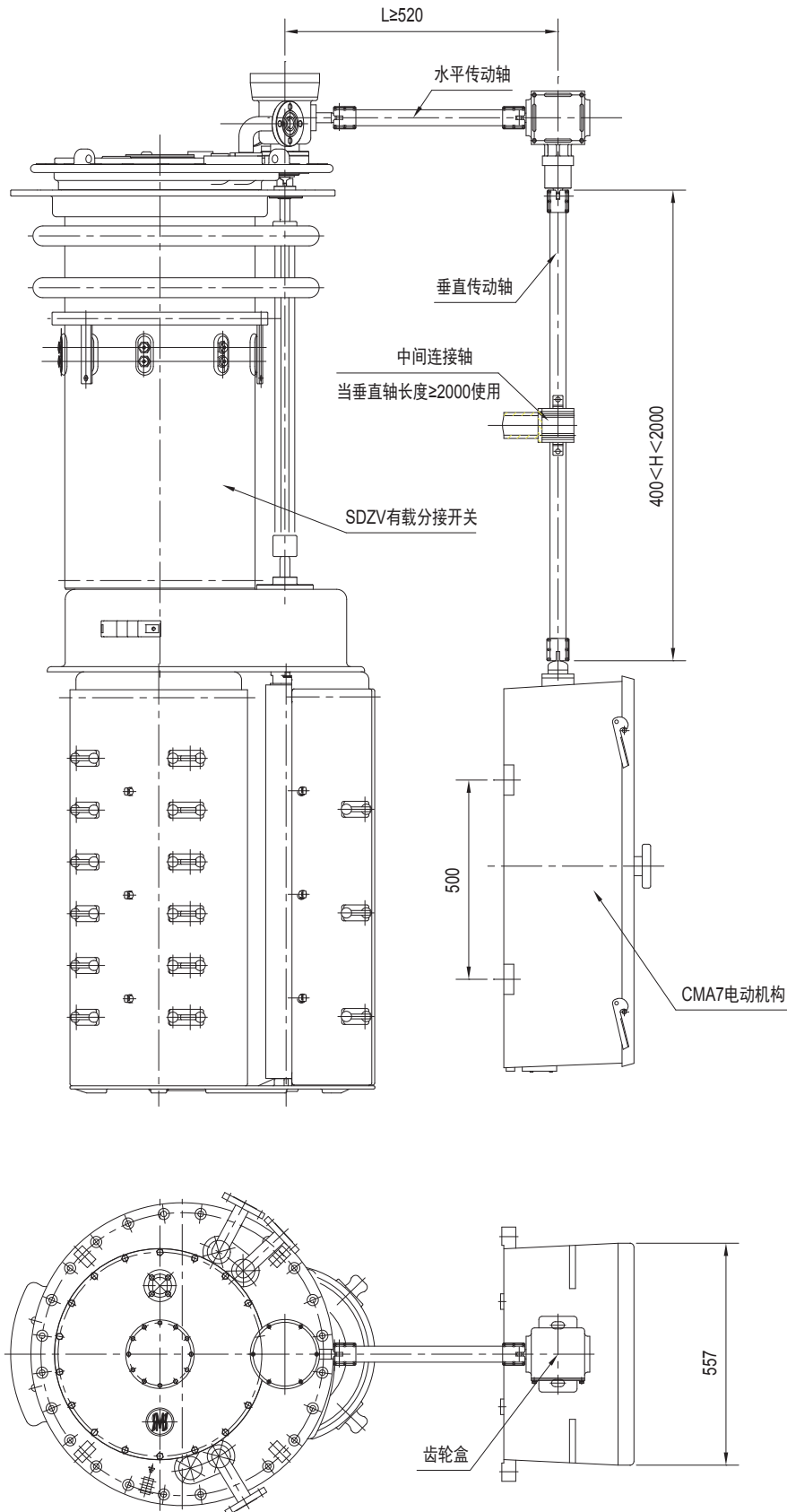
附图 9 SDZV 分接开关与 CMA7 电动机构连接布置图
