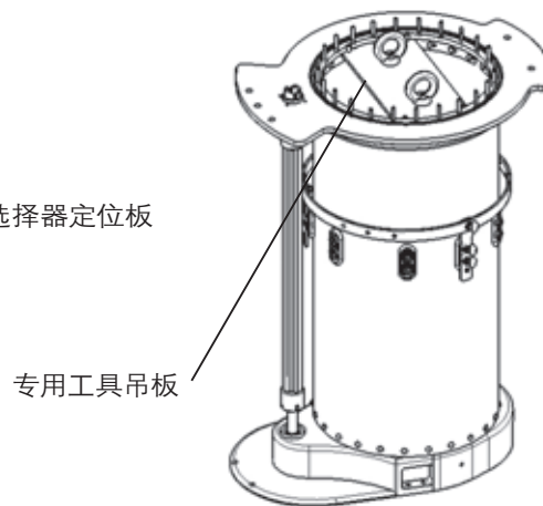
图-10 油室起吊环
