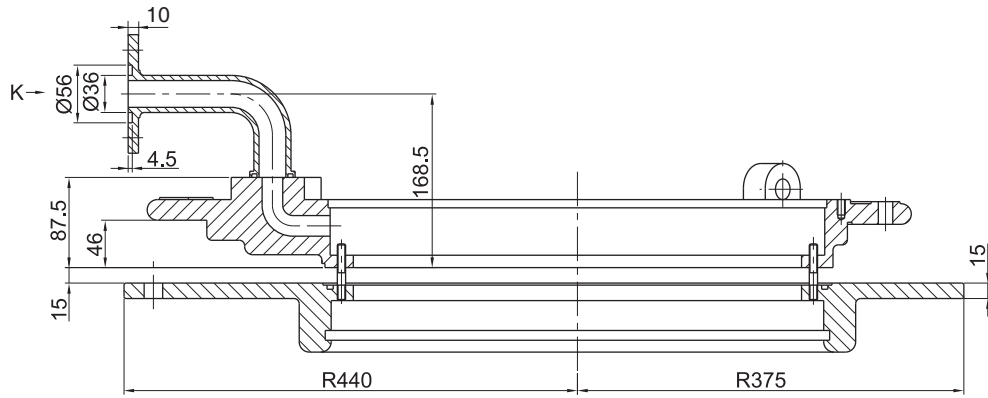
附图 1 SDZV 有载分接开关变压器安装法兰尺寸
