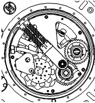
图 11 储能机构
