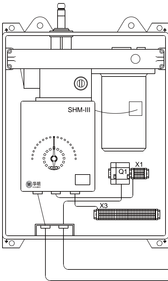
X3端子说明：一、一对应信号输出
